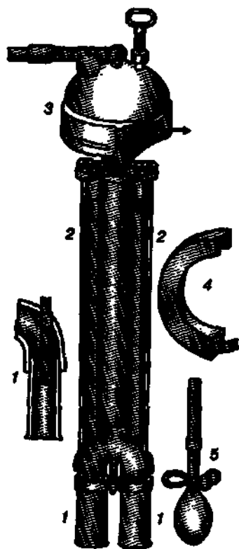
Рис. 2.6. Психрометр Асмана:
