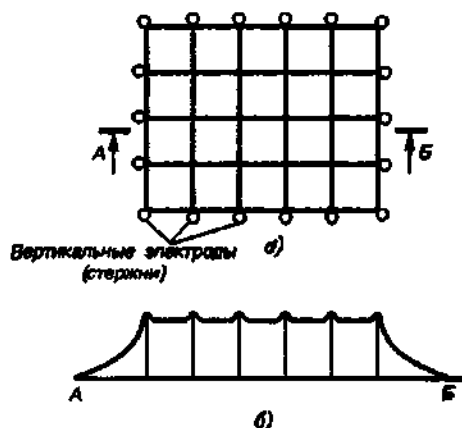
Рис. 7.8. Заземлитель с выравниваем потенциалов внутри контура (сетка):
