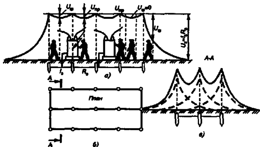
Рис. 7.7. Контурное заземление:
