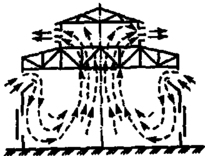
Рис. 2.1. Схемы аэрации в помещении
