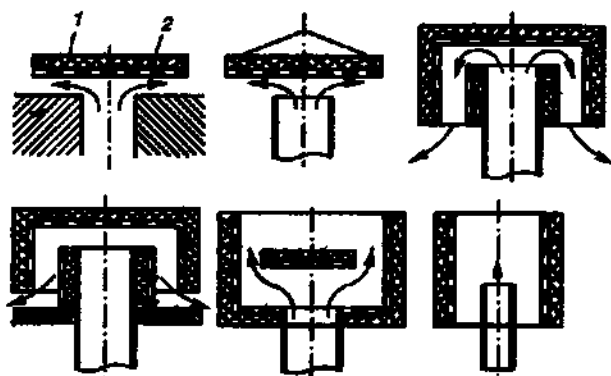
Рис. 7.24. Экранированные глушители:
