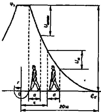
Рис. 7.4. Напряжение шага
