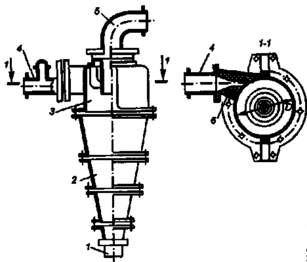
Рис. 7.52. Напорный гидроциклон:
