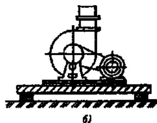
Рис. 7.14. Установка агрегатов на виброгасящем основании:
