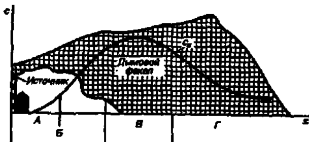
Рис. 5.1. Распределение концентраций вредных веществ в атмосфере у земной поверхности от организованного высокого источника выбросов:
