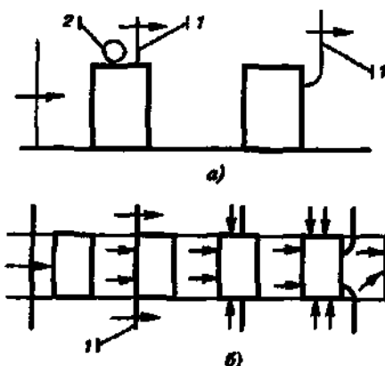
Рис. 9.3. Взаимодействие воздушной ударной волны с плоским препятствием:
