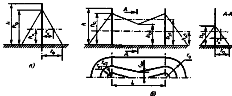
Рис. 9.5. Некоторые типы молниеотводов:
