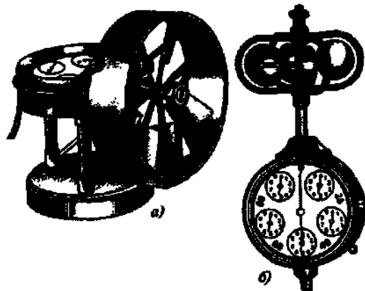
Рис. 2.7. Анемометры:
