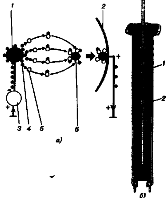
Рис. 7.44. Схема электростатического осаждения частиц (а) (1 — коронирующий электрод; 2 — осадительный электрод; 3 — агрегат электропитания; 4 — электрон; 5 — молекула газа; 6 — осаждаемая частица) и электродная пара с трубчатым осадительным электродом (б) (1 — трубчатый осадительный электрод; 2 — коронирующий электрод)
