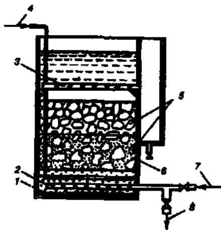
Рис. 7.53. Карбисно-засыпной фильтр:
