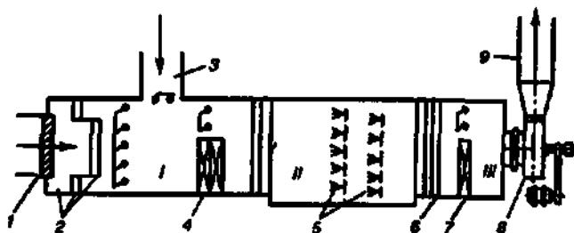
Рис. 2.5. Схемы кондиционера:
